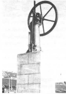
Modell des Ottomotors von Nikolaus August Otto auf dem Ottoplatz am Deutzer Bahnhof
